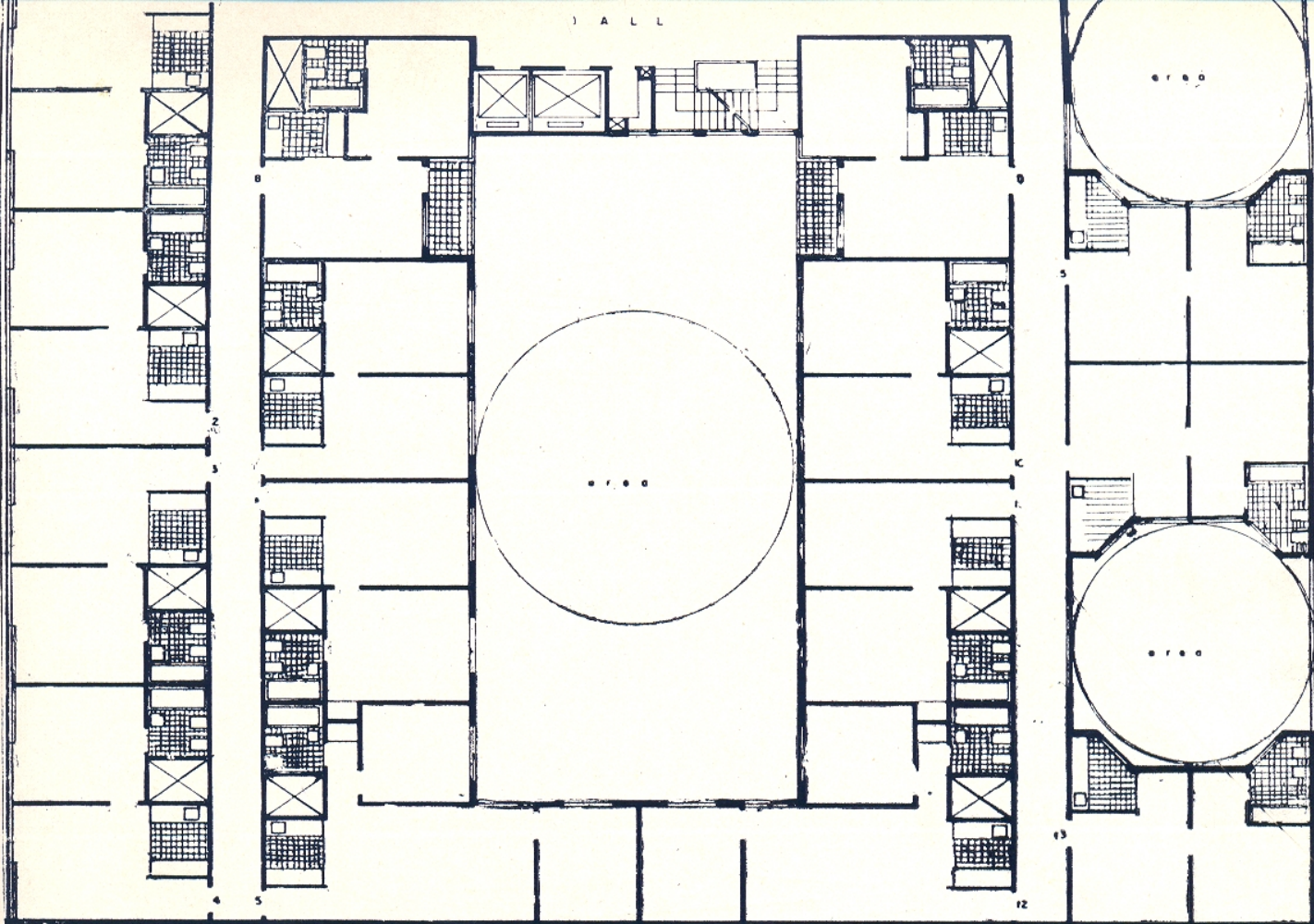
ANDAR TIPO
